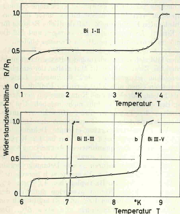
Abb. 8 und 9. Übergangskurven von Wismut. 8 bei 25,4 kbar. 9a bei 27 kbar; 9b bei 78 kbar
